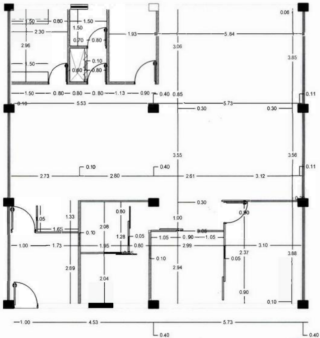
PLANTA ARQUITECTONICA DIMENSIONADA PROPUESTA DEPARTAMENTO DE JURIDICA MSP
